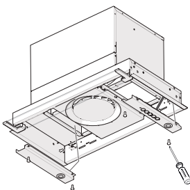
2) irrota ruuvit 4x (M4x10)
