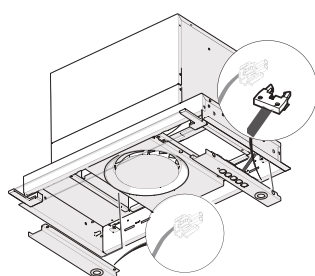
3) Atjunkite kabelius
