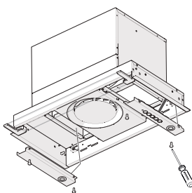
2) Fjern skruene 4x (M4x10)
