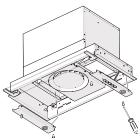
2) Fjern skruerne 4x (M4x10)
