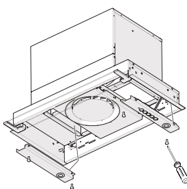
2) Išimkite 4x varžtus (M4x10)
