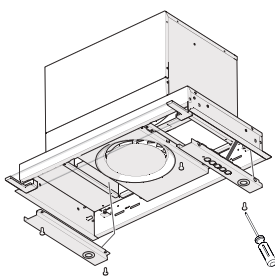
2) Ta bort skruvarna 4x (M4x10)
