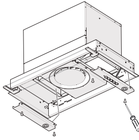
2) 4x vidalarını çıkartınız (M4x10)
