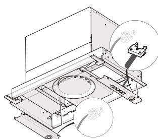
3) odpojte kabely
