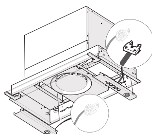
3) odklopite kable
