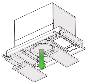
1) odstranite maščobne filtre
