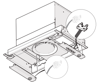
3) kablo bağlantısını kesiniz
